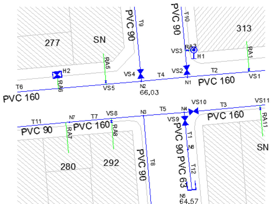
Figura 1 – Representação esquemática da rede – troços de conduta, nós e órgãos constituintes devidamente georreferenciados e codificados
